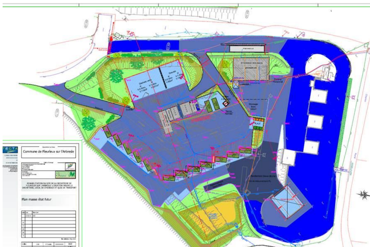
Plan : nouvelle déchetterie de Fleury sur l'Arbresle
